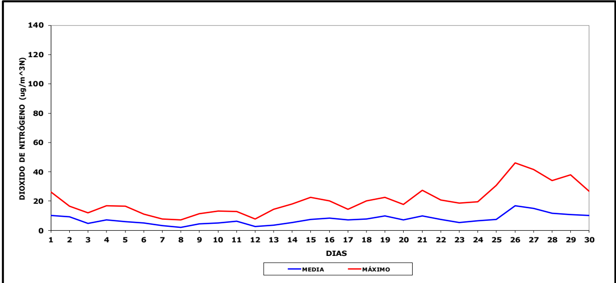
Gráfico N° 7 Concentración Dióxido de Nitrógeno Maitencillo, Junio 2024
