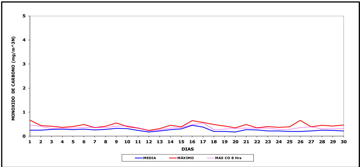
Gráfico N° 5 Concentración de Monóxido de Carbono, Junio 2024
