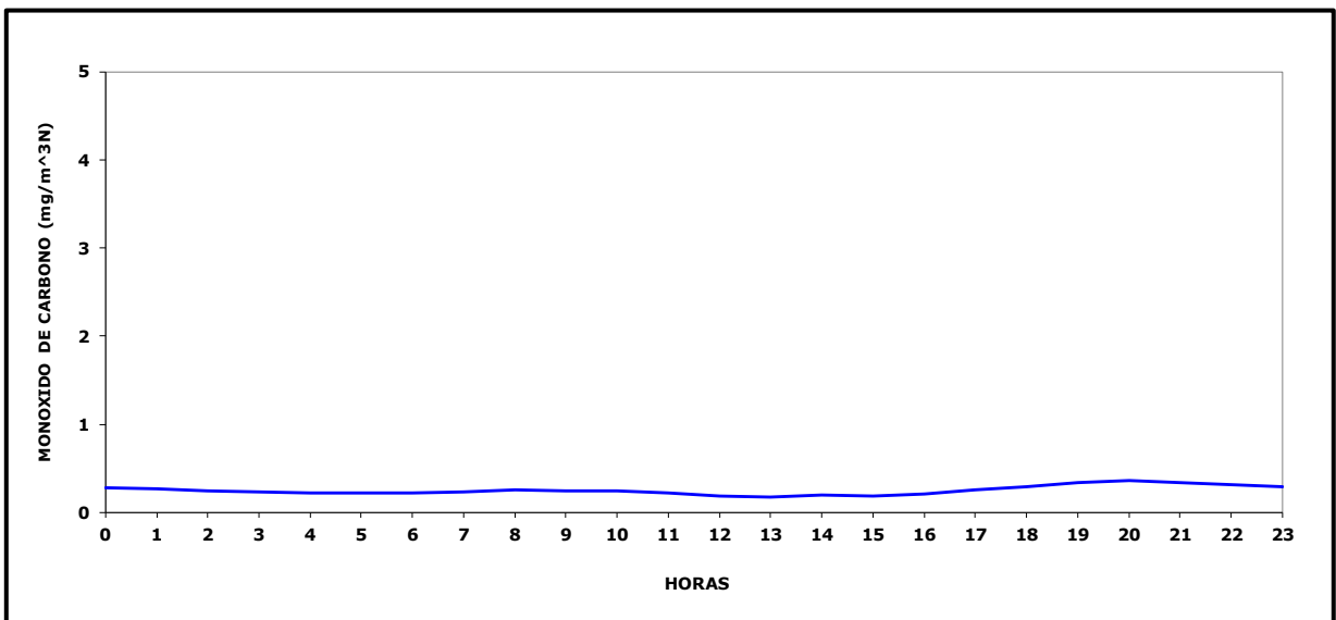
Gráfico N° 6 Ciclo Diario Monóxido de Carbono, Junio 2024
