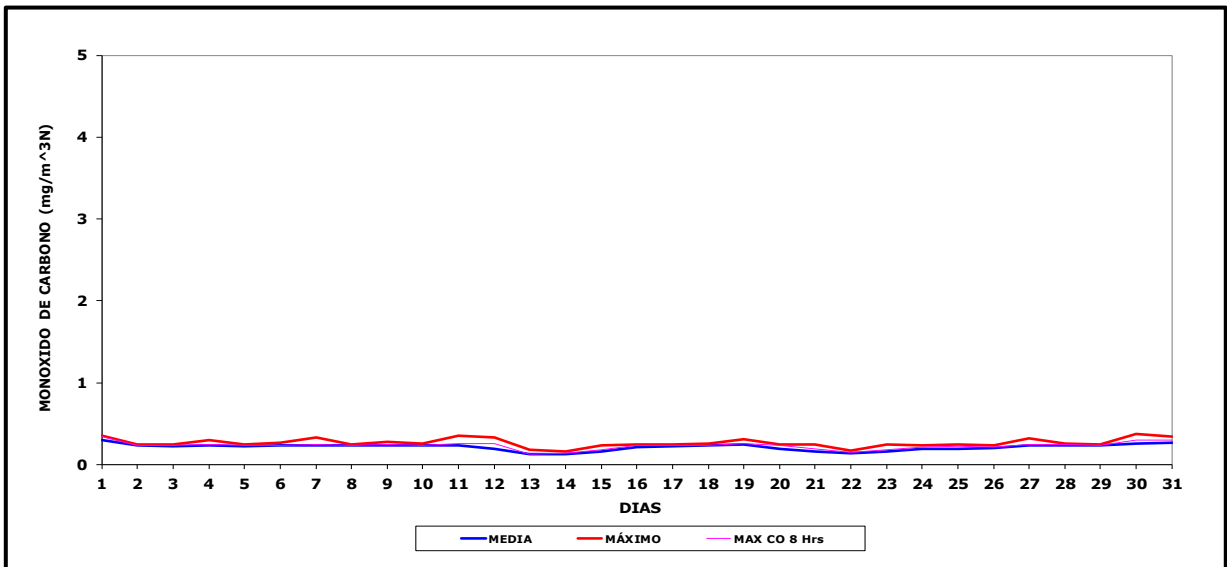
Gráfico N° 5 Concentración de Monóxido de Carbono, Marzo 2024
