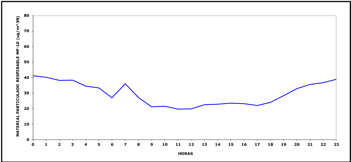
Gráfico N° 2 Ciclo Diario MP-10 Estación Maitencillo, Marzo 2024
