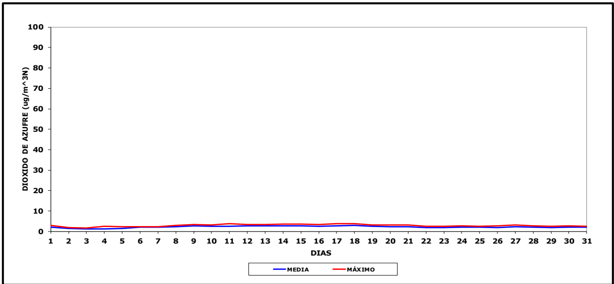
Gráfico N° 3 Concentración de Dióxido de Azufre, Marzo 2024
