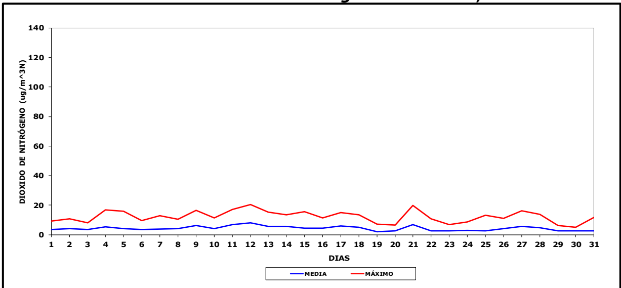
Gráfico N° 7 Concentración Dióxido de Nitrógeno Maitencillo, Marzo 2024
