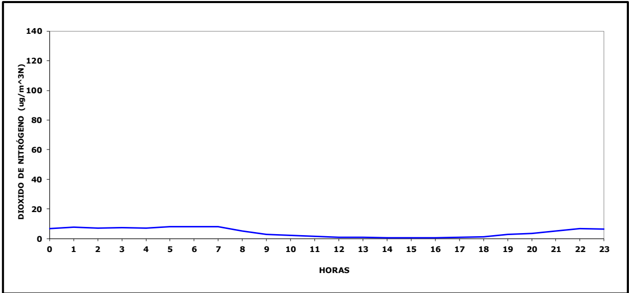
Gráfico N° 8 Ciclo Diario Dióxido de Nitrógeno Maitencillo, Marzo 2024
