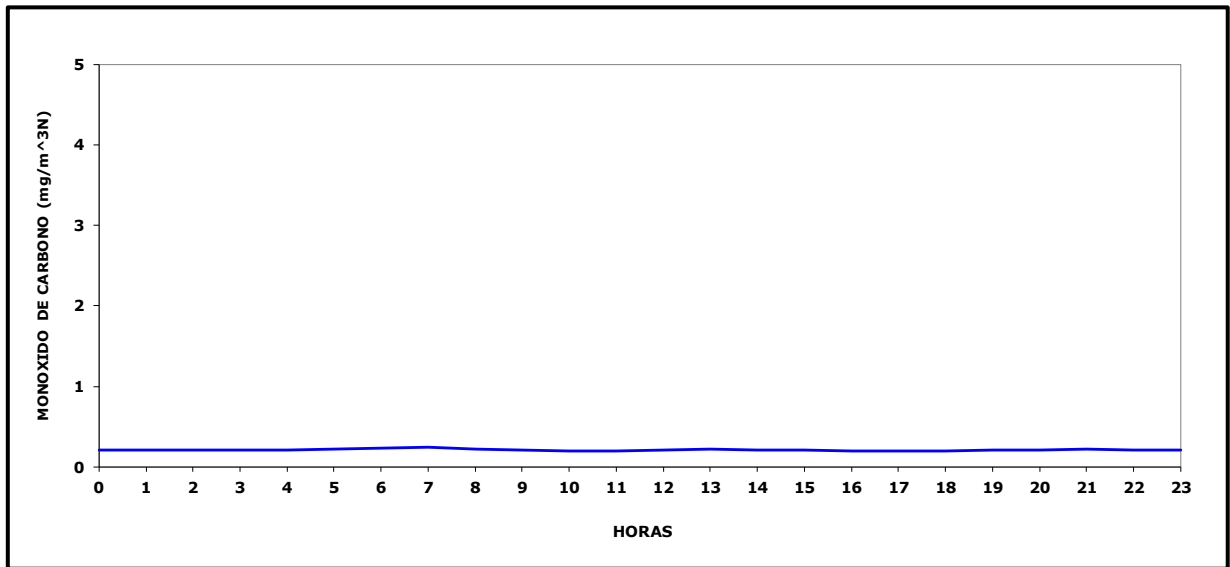
Gráfico N° 6 Ciclo Diario Monóxido de Carbono, Marzo 2024
