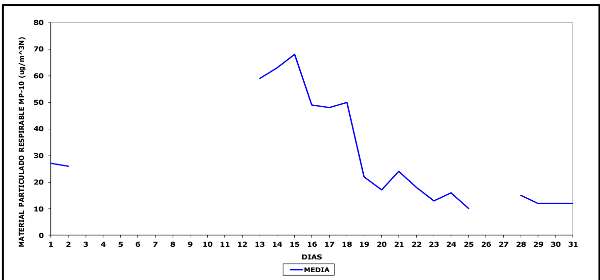
Gráfico N° 1 Concentración de MP-10 Estación Maitencillo h , Marzo 2024
