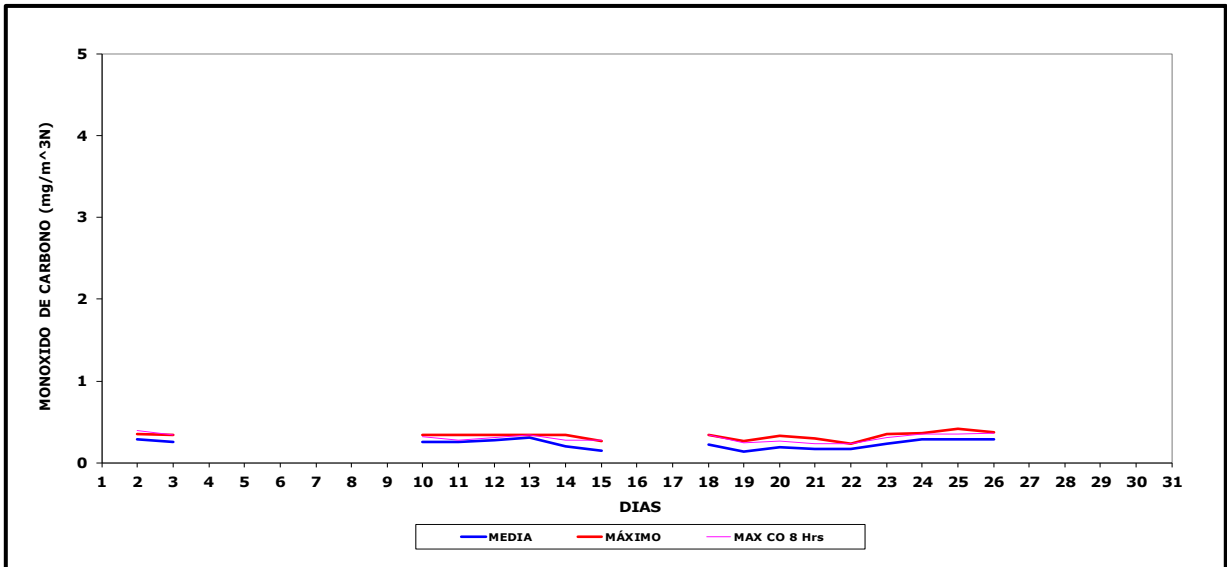
Gráfico N° 5 Concentración de Monóxido de Carbono i , Enero 2024
