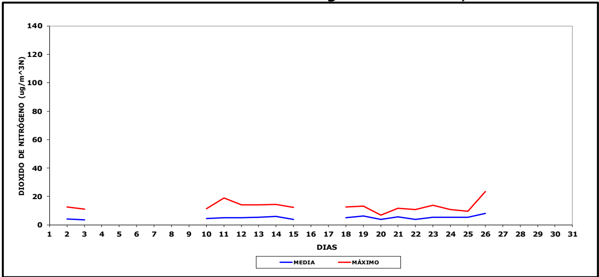
Gráfico N° 7 Concentración Dióxido de Nitrógeno Maitencillo j , Enero 2024
