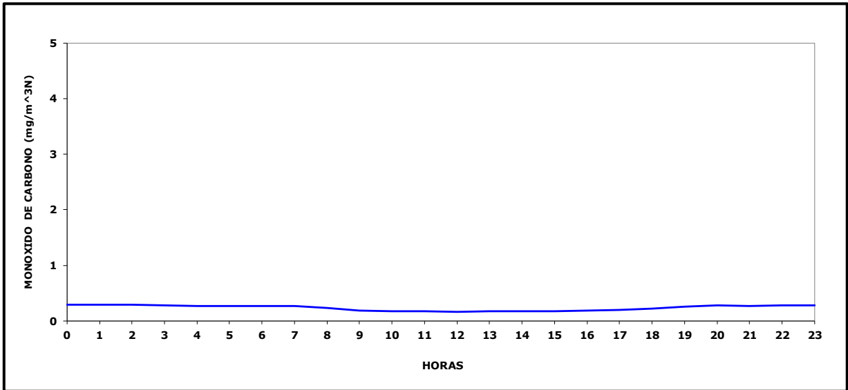
Gráfico N° 6 Ciclo Diario Monóxido de Carbono, Enero 2024
