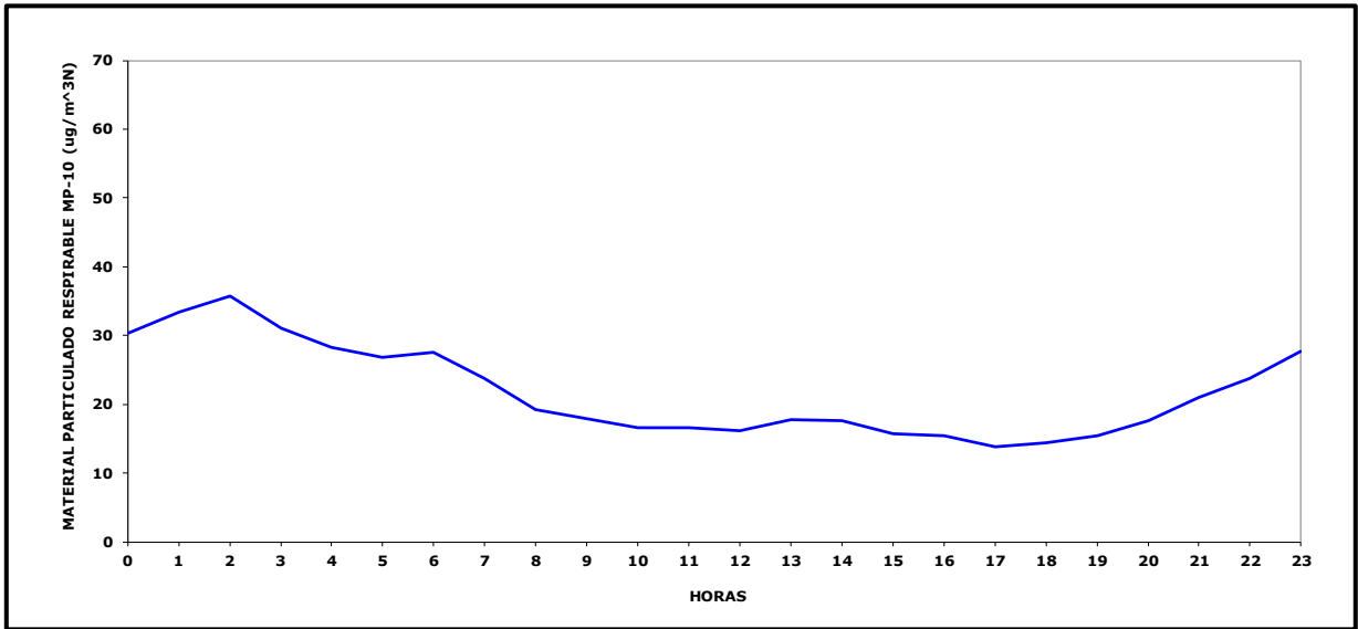
Gráfico N° 2 Ciclo Diario MP-10 Estación Maitencillo, Enero 2024
