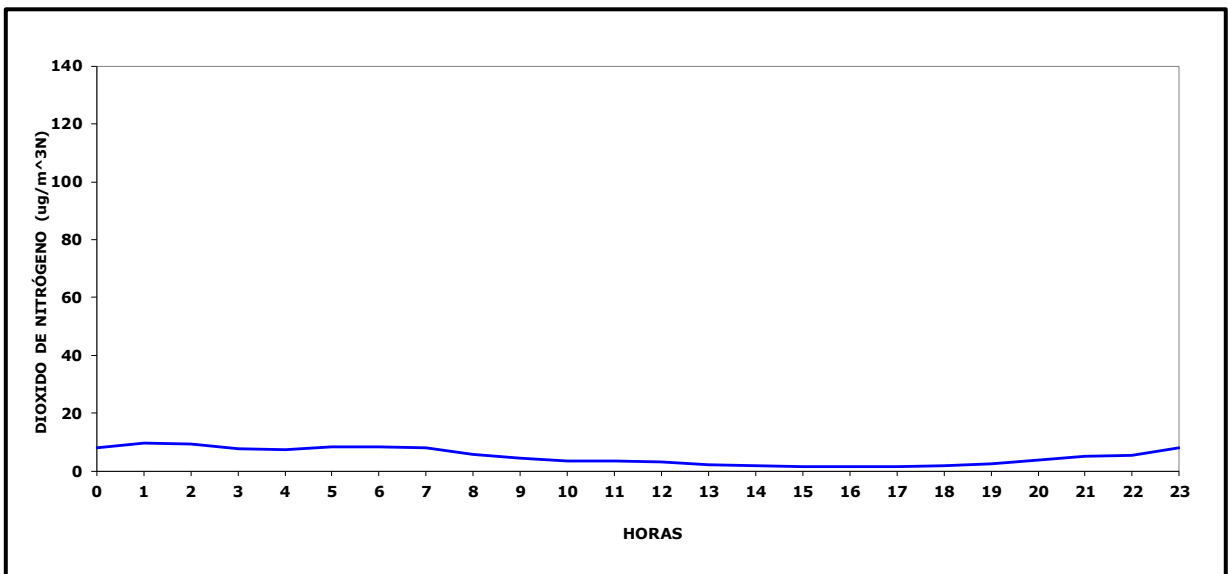
Gráfico N° 8 Ciclo Diario Dióxido de Nitrógeno Maitencillo, Enero 2024
