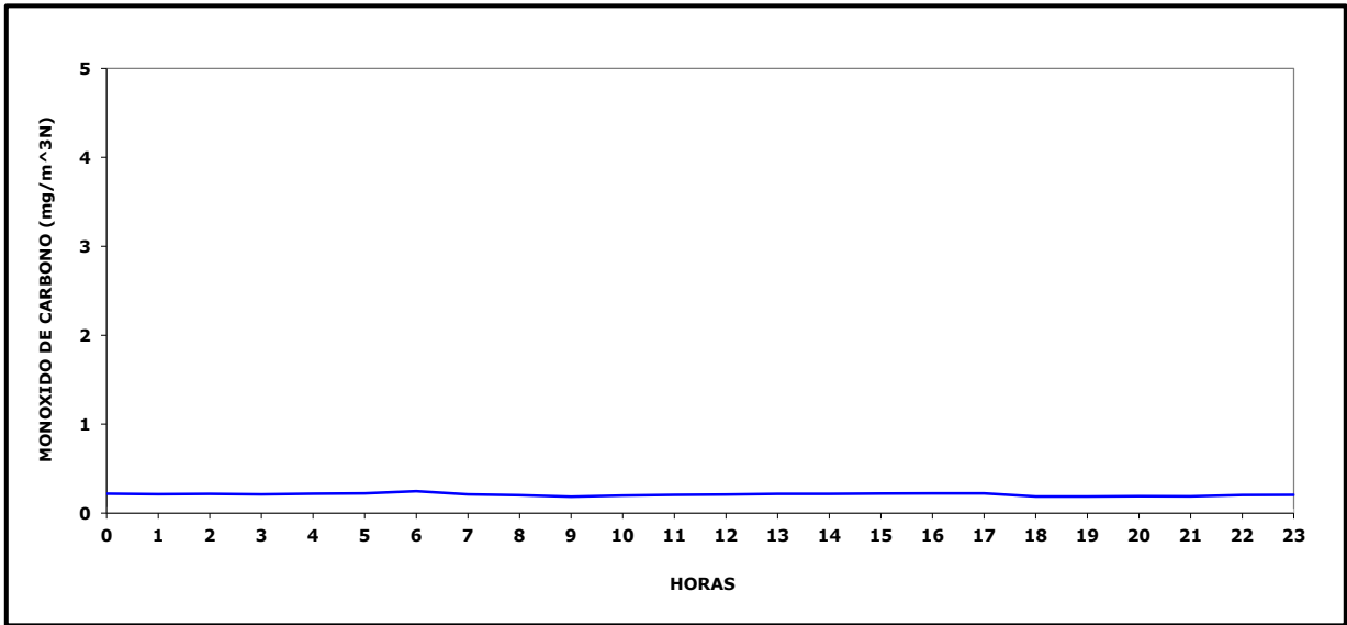
Gráfico N° 6 Ciclo Diario Monóxido de Carbono, Noviembre 2022
