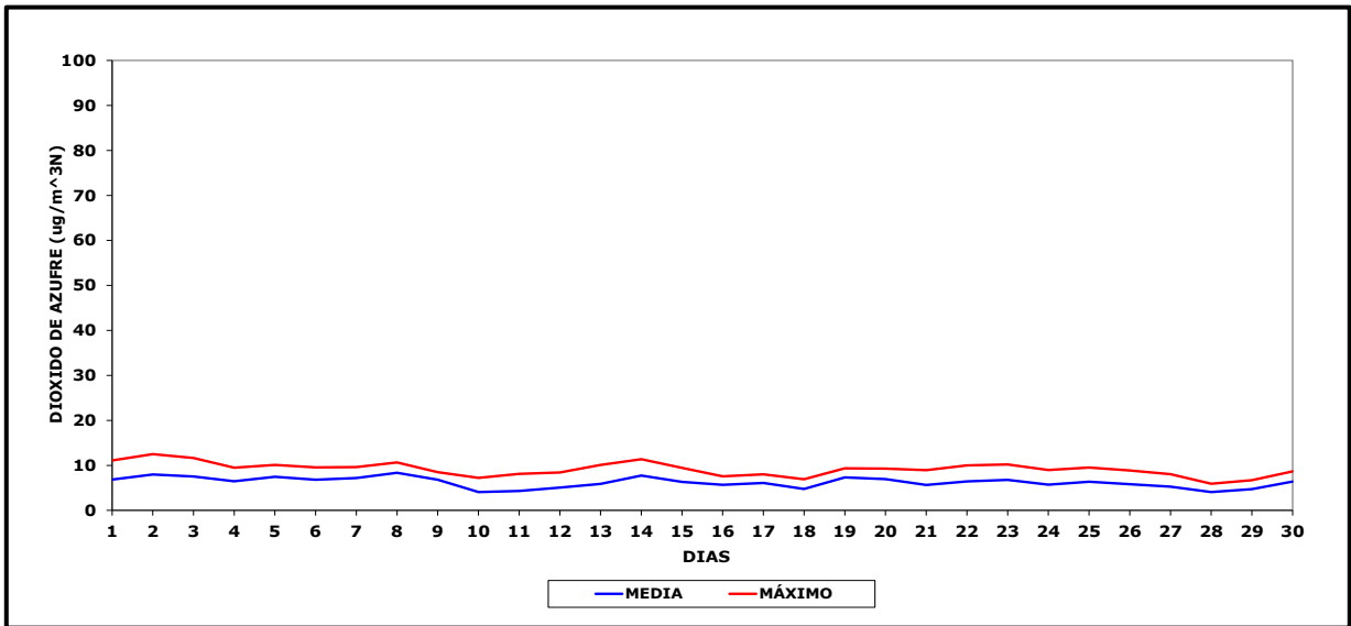
Gráfico N° 3 Concentración de Dióxido de Azufre, Noviembre 2022
