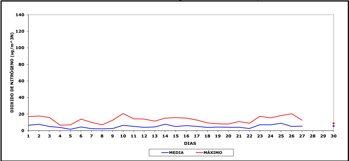
Gráfico N° 7 Concentración Dióxido de Nitrógeno Maitencillo f , Noviembre 2022
