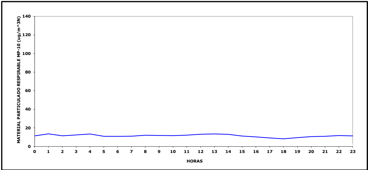
Gráfico N° 2 Ciclo Diario MP-10 Estación Maitencillo, Noviembre 2022
