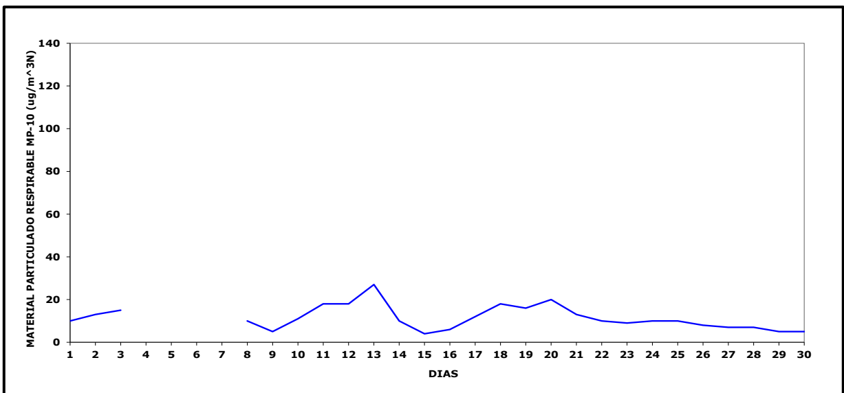
Gráfico N° 1 Concentración de MP-10 Estación Maitencillo d , Noviembre 2022
