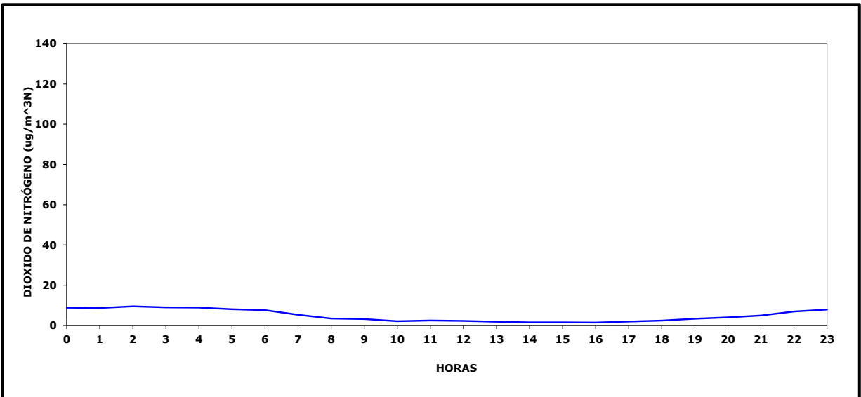
Gráfico N° 8 Ciclo Diario Dióxido de Nitrógeno Maitencillo, Noviembre 2022
