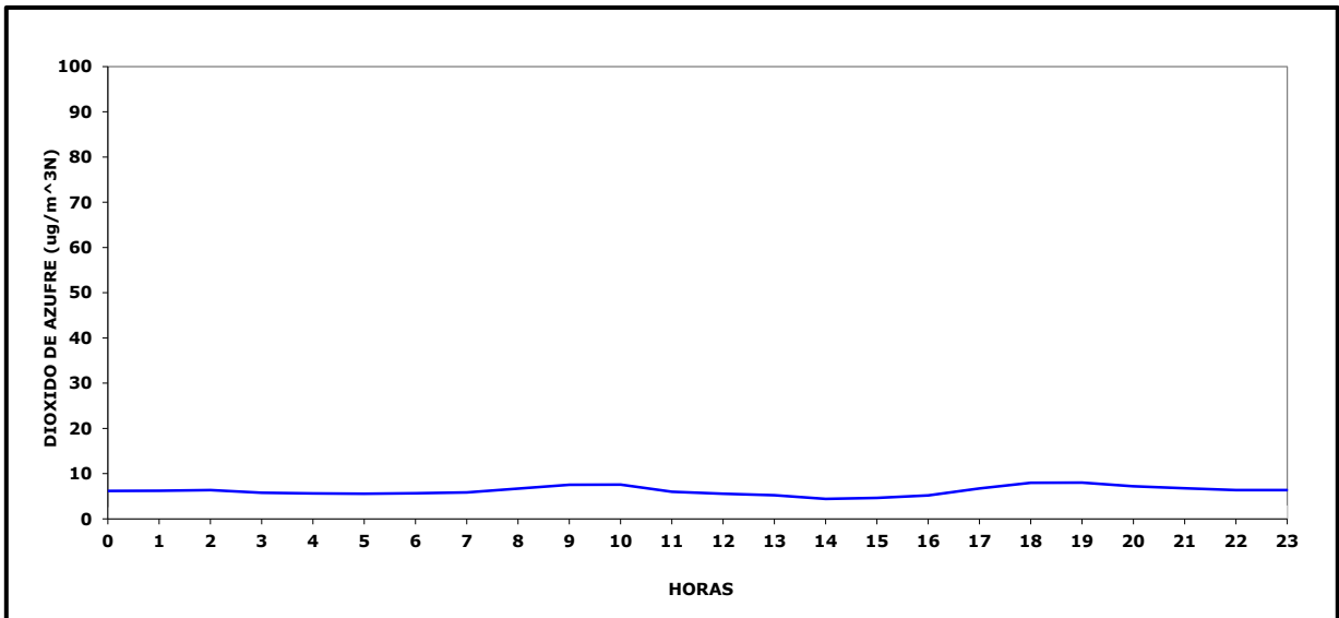
Gráfico N° 4 Ciclo Diario Dióxido de Azufre, Noviembre 2022
