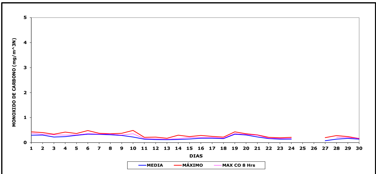
Gráfico N° 5 Concentración de Monóxido de Carbono e , Noviembre 2022
