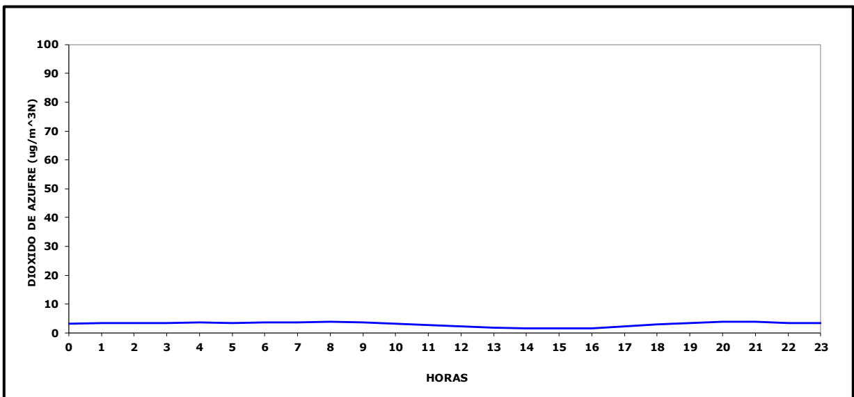
Gráfico N° 4 Ciclo Diario Dióxido de Azufre, Julio 2023
