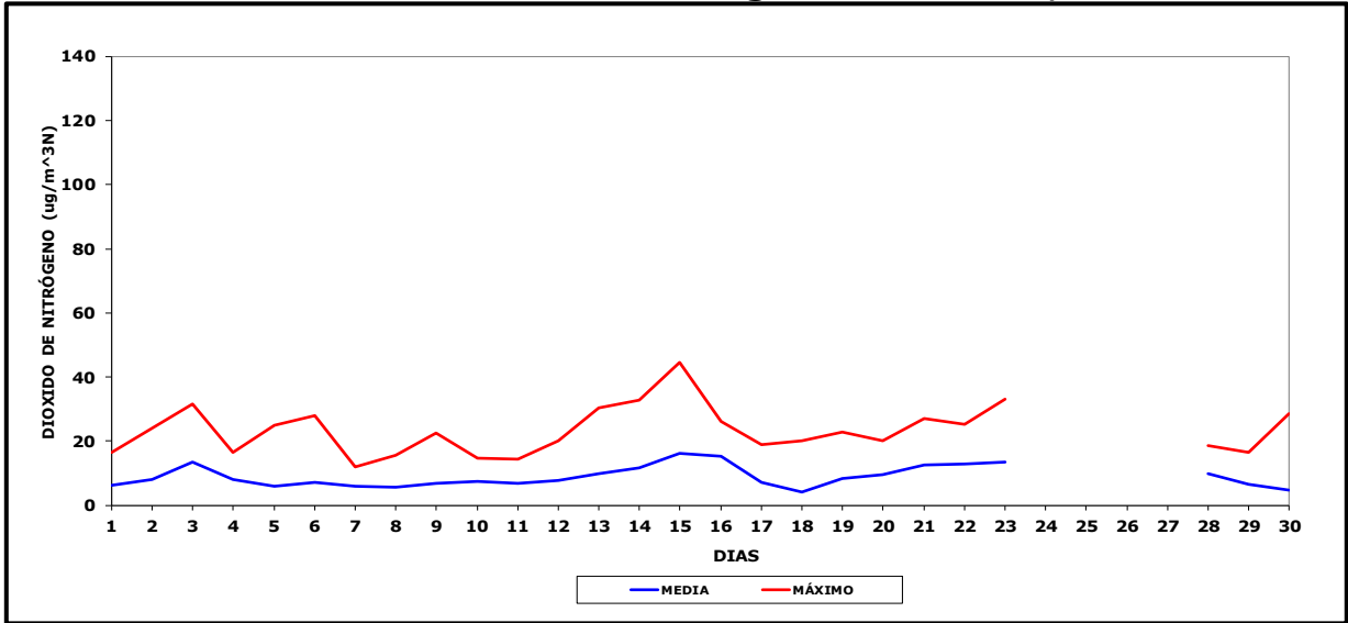
Gráfico N° 7 Concentración Dióxido de Nitrógeno Maitencillo j , Julio 2023
