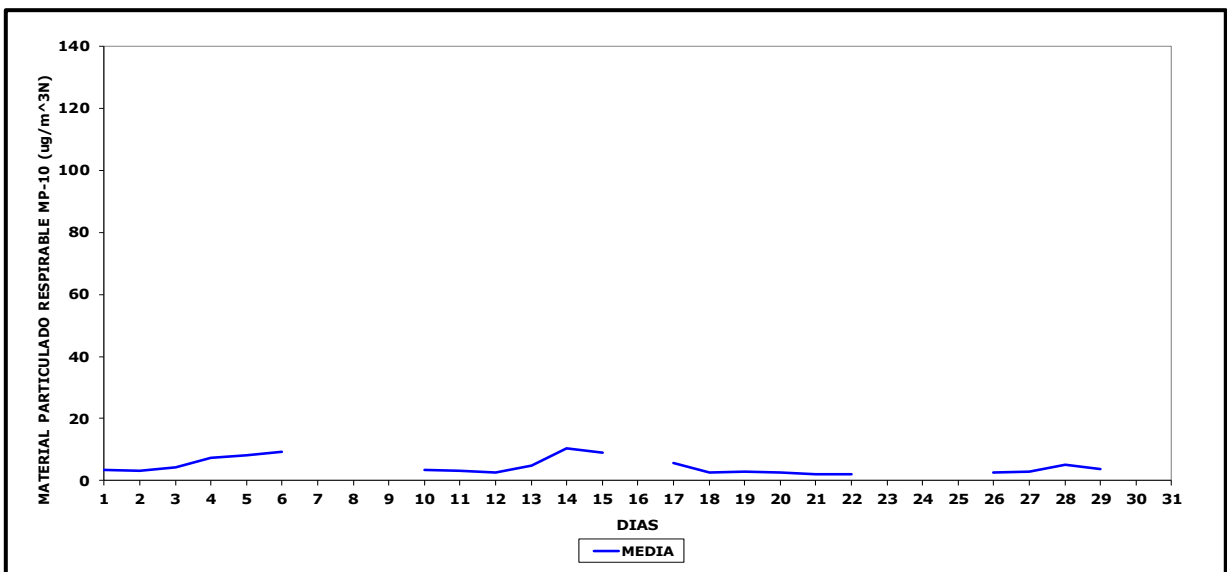
Gráfico N° 1 Concentración de MP-10 Estación Maitencillo 9 , Julio 2023
