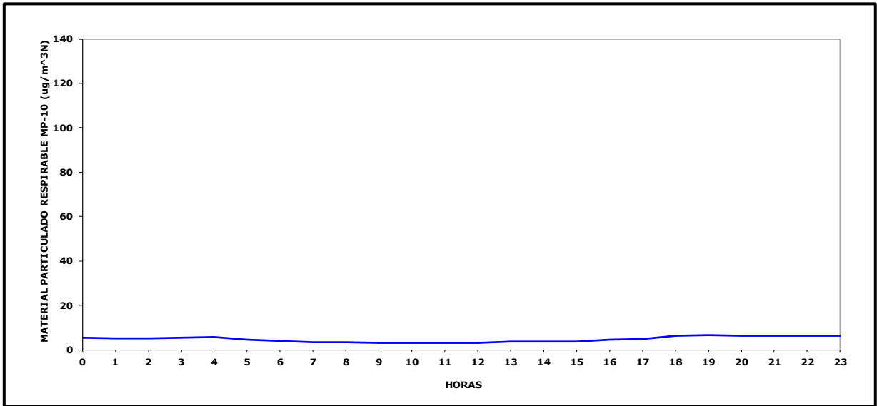
Gráfico N° 2 Ciclo Diario MP-10 Estación Maitencillo, Julio 2023
