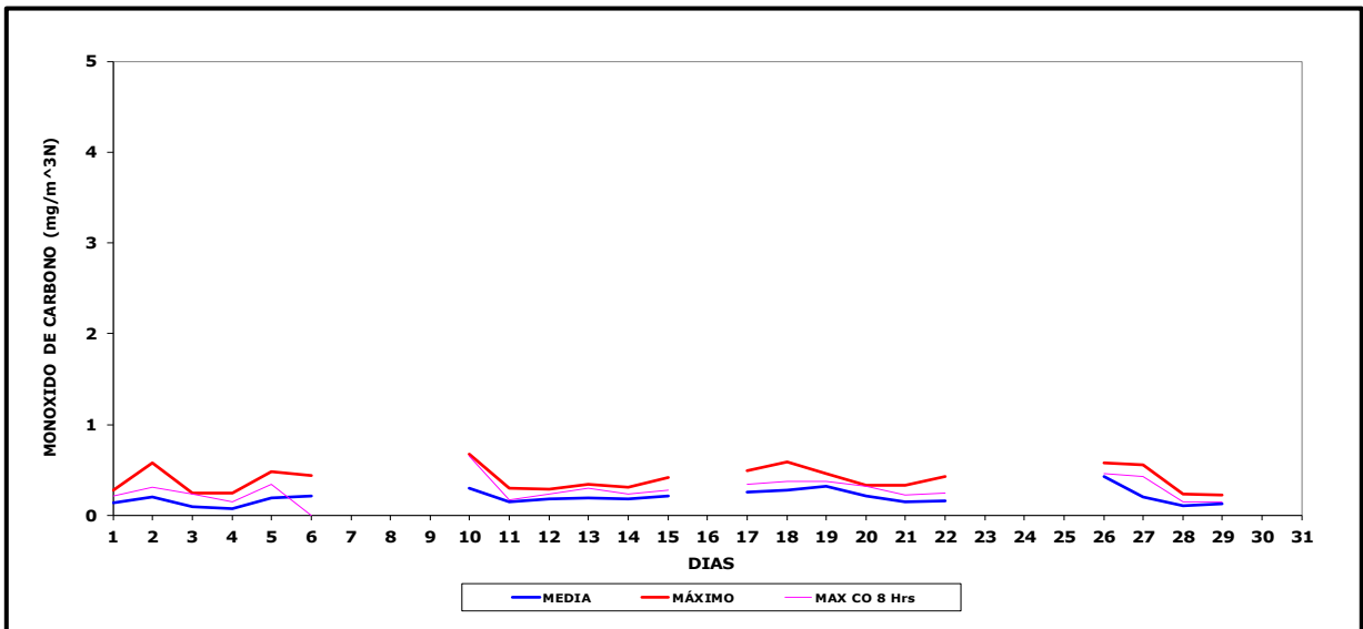
Gráfico N° 5 Concentración de Monóxido de Carbono i , Julio 2023
