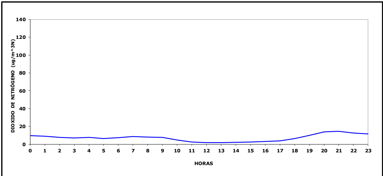
Gráfico N° 8 Ciclo Diario Dióxido de Nitrógeno Maitencillo, Julio 2023
