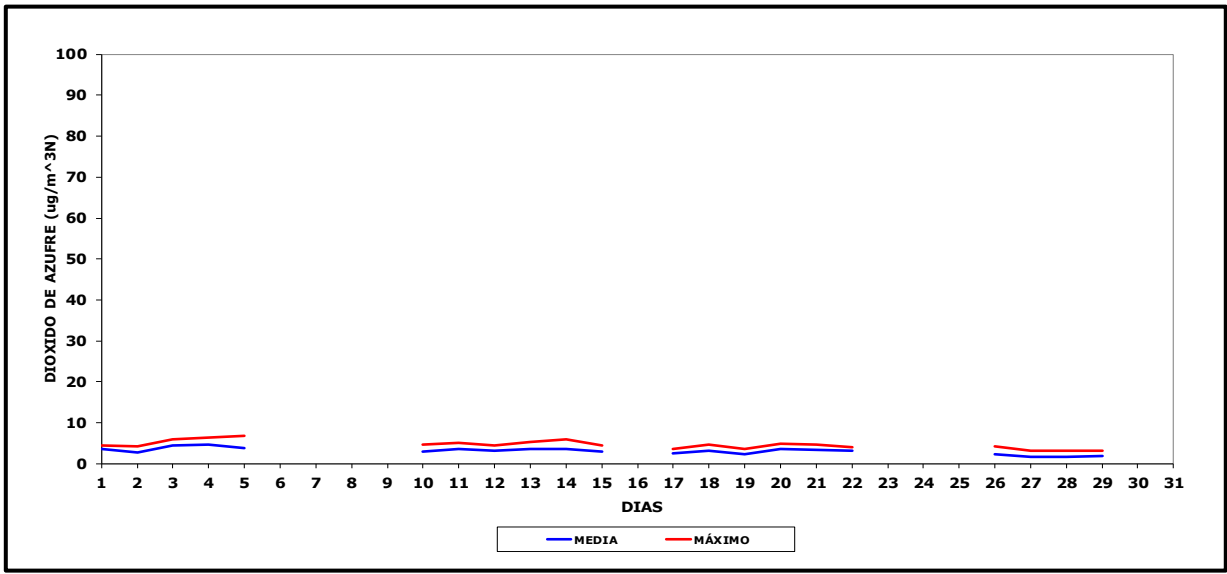
Gráfico N° 3 Concentración de Dióxido de Azufre h , Julio 2023
