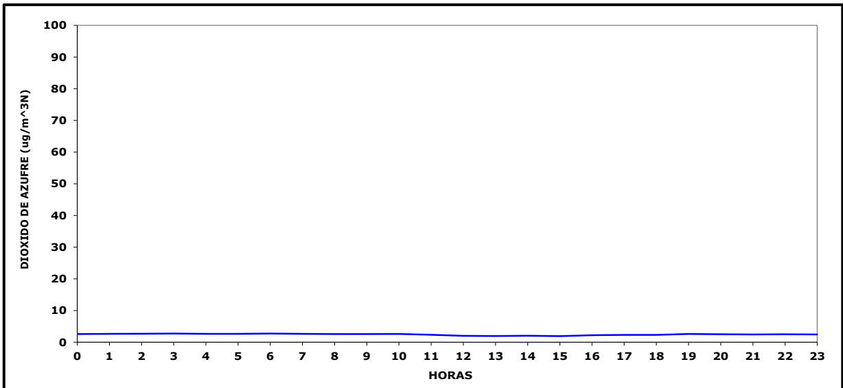
Gráfico N° 4 Ciclo Diario Dióxido de Azufre, Marzo 2023
