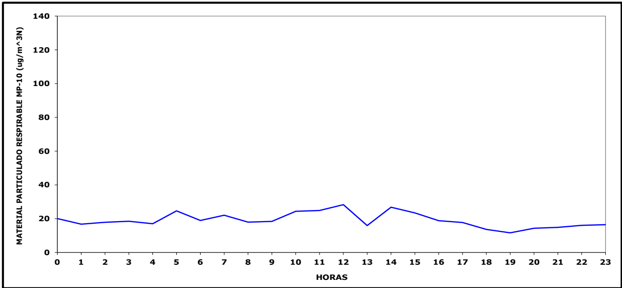
Gráfico N° 2 Ciclo Diario MP-10 Estación Maitencillo, Marzo 2023
