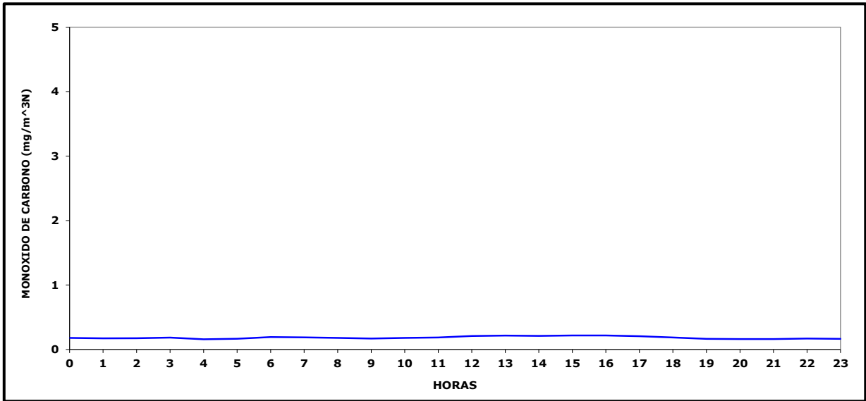
Gráfico N° 6 Ciclo Diario Monóxido de Carbono, Marzo 2023
