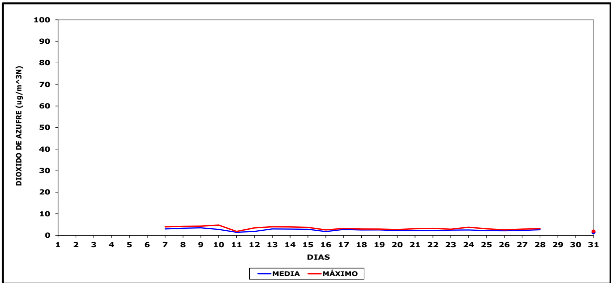
Gráfico N° 3 Concentración de Dióxido de Azufre 9 , Marzo 2023
