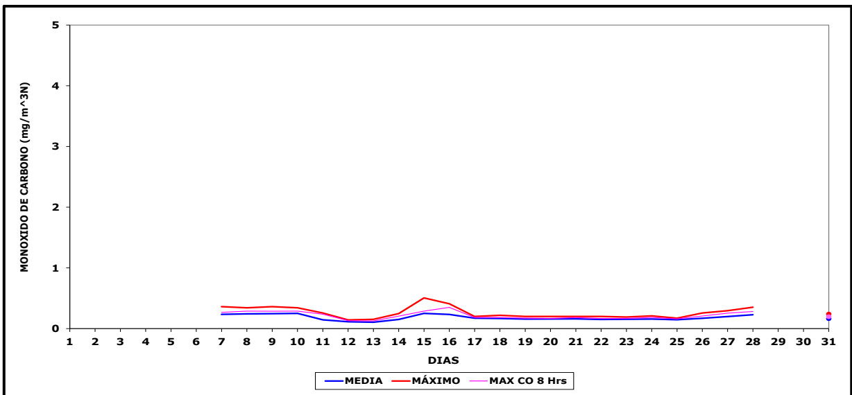
Gráfico N° 5 Concentración de Monóxido de Carbono, Marzo 2023
