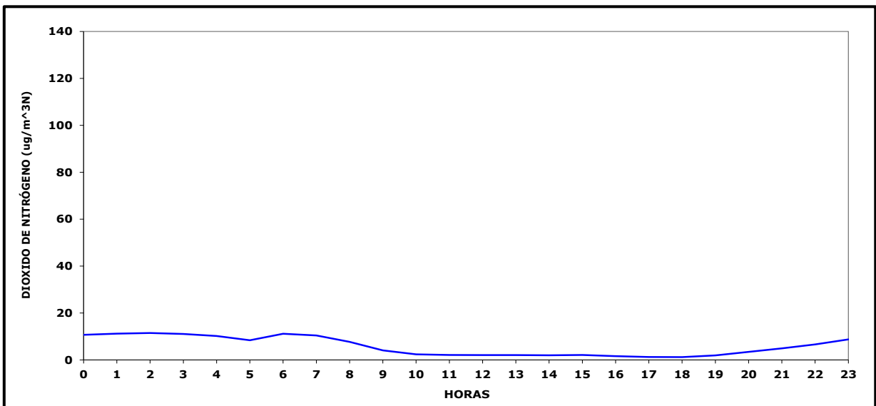
Gráfico N° 8 Ciclo Diario Dióxido de Nitrógeno Maitencillo, Marzo 2023
