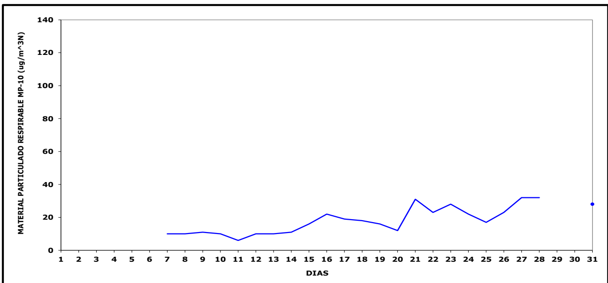
Gráfico N° 1 Concentración de MP-10 Estación Maitencillo f , Marzo 2023
