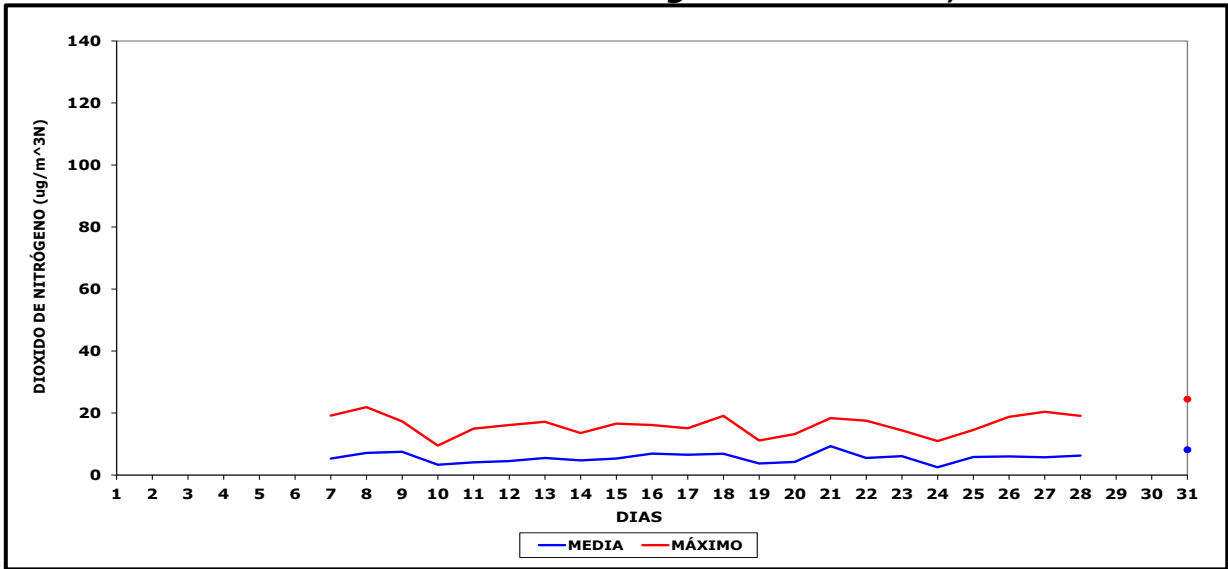
Gráfico N° 7 Concentración Dióxido de Nitrógeno Maitencillo h , Marzo 2023
