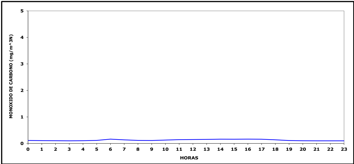
Gráfico N° 6 Ciclo Diario Monóxido de Carbono, Enero 2023
