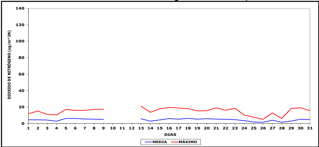
Gráfico N° 7 Concentración Dióxido de Nitrógeno Maitencillo i , Enero 2023
