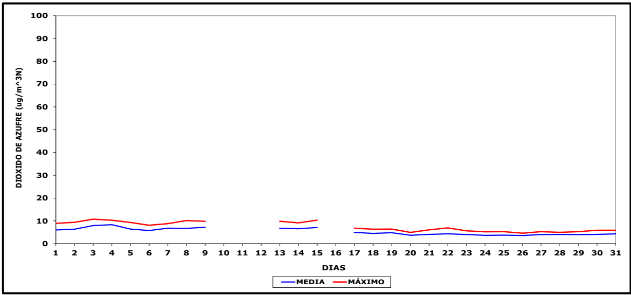
Gráfico N° 3 Concentración de Dióxido de Azufre 9 , Enero 2023
